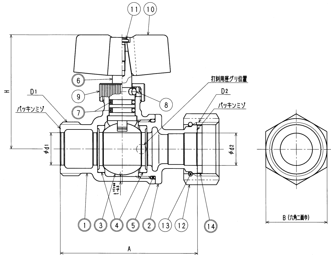
寸法表
